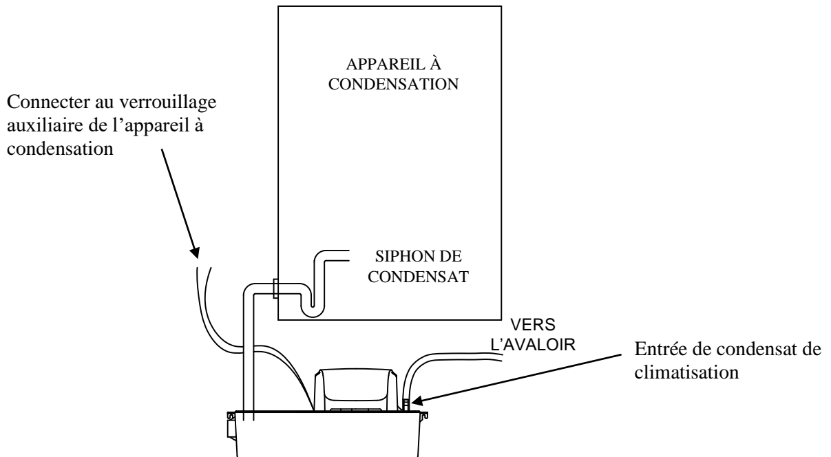
Figure 4 – Schéma d'installation du Bac De Neutralisation
